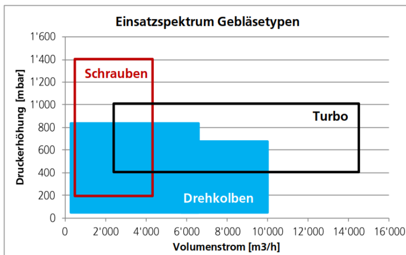
Abbildung 7: Einsatzbereich Gebläsetypen
