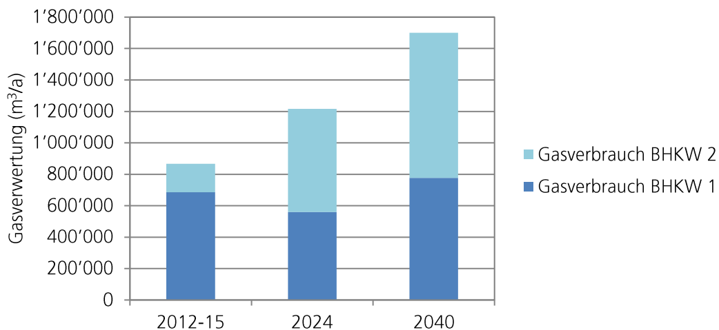
Abbildung 3: Gasverwertung in den BHKWs bis Ausbauziel 2040, Quelle: Konzept BHKW [3]
